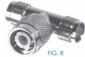
FIG. 8 RFT-1228
